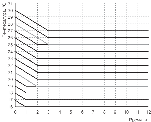
Кривые изменения температуры в режиме сна для режима обогрева
